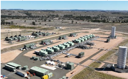
〈신규 가스처리시설 1/2호기 전경〉
